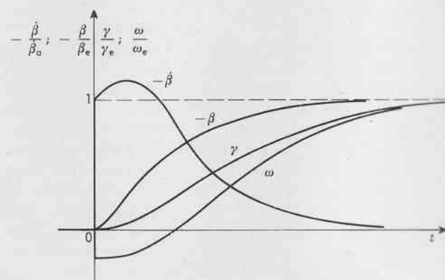
Bild 2. Übergangsfunktionen für \beta , \dot{\beta} , \gamma und \omega bei einem Lenkwinkelsprung \delta = \delta_0 für t = 0 .
