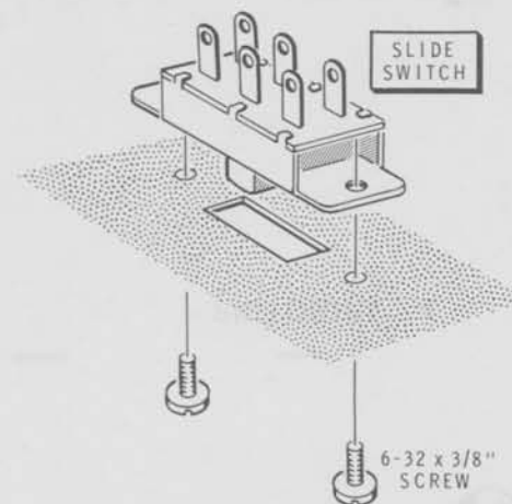
Detail 2-3E
