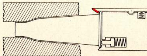
Extracteur et éjecteur (à la fin de la fermeture).
