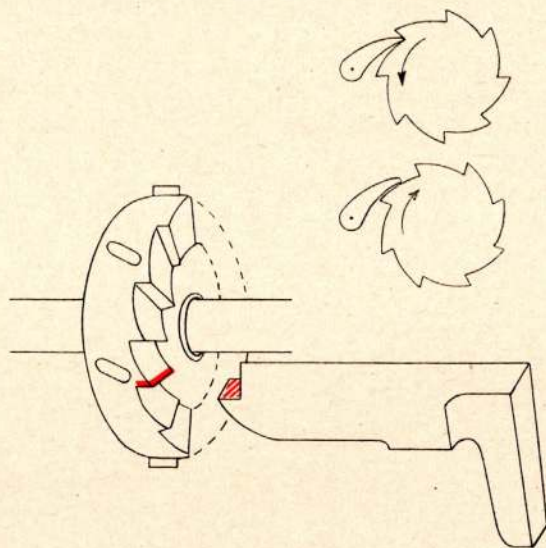
Cliquet et rochet de l'entraîneur.
