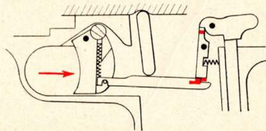
Pendant l'armé (avant l'abandon de la détente).
