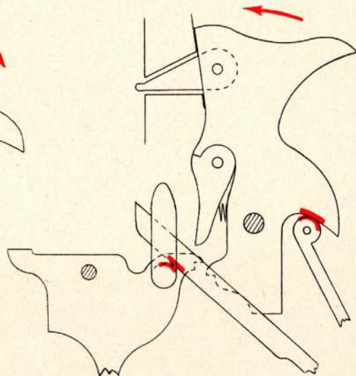
PERCUSSION (Saillie du percuteur)
