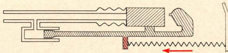
Piston en avant.
