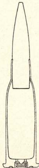
Cartouche modèle 1886 D (am)
