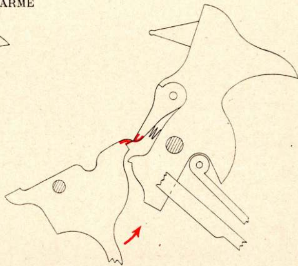
Fin de l'armé (tir continu).
