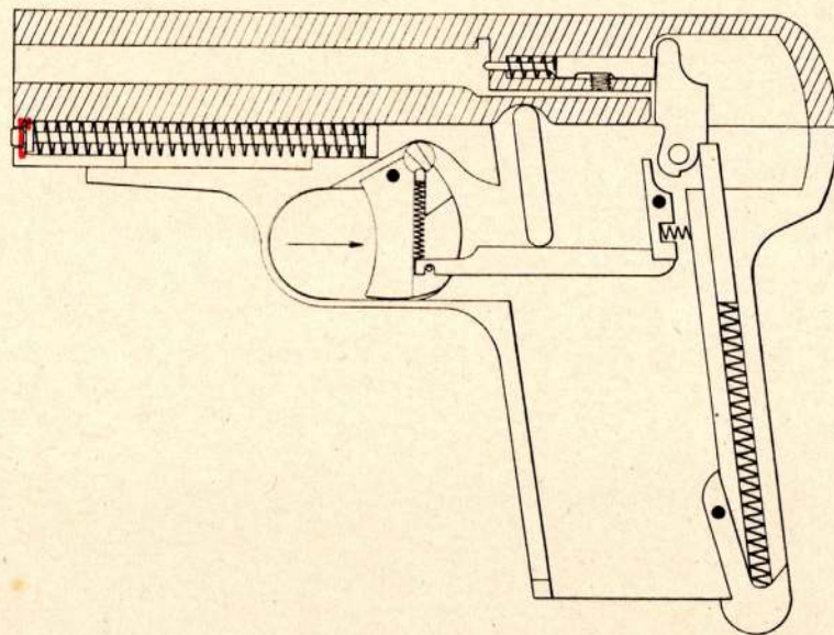
COUPE DU PISTOLET (chien à l'abattu).
