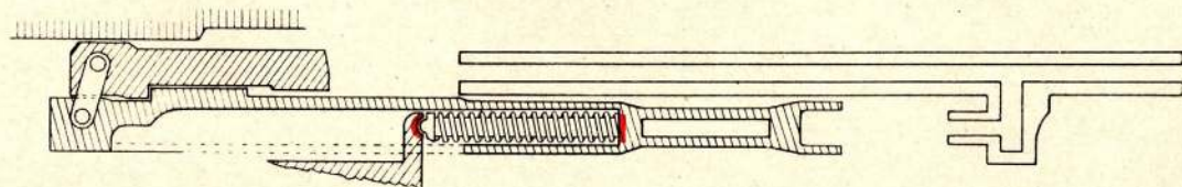
Piston en arrière.
