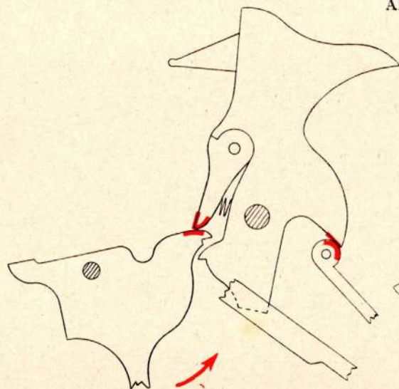
Début de l'armé (tir continu).
