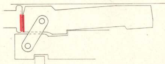
Ouverture ( Position extrême de la culasse ).
