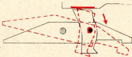
Levier de gâchette et mentonnet.
