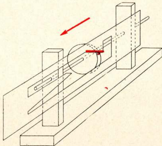
b) Petite came (O).
