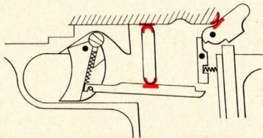
Pendant l'armé (détente pressée ou non)
