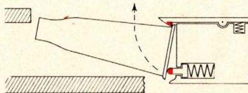
Extracteur et éjecteur (à la fin de la fermeture).
