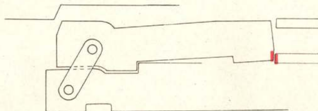
Ouverture ( Position extrême de la culasse ).
