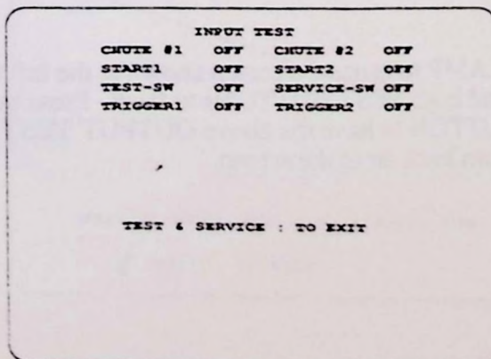
FIG. 8.6 INPUT TEST
