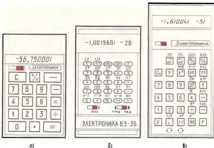
Рис. 4. Микрокалькуляторы типа:
