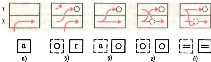
Рис. 6. Схемы работы операционного стека арифметического микрокалькулятора
