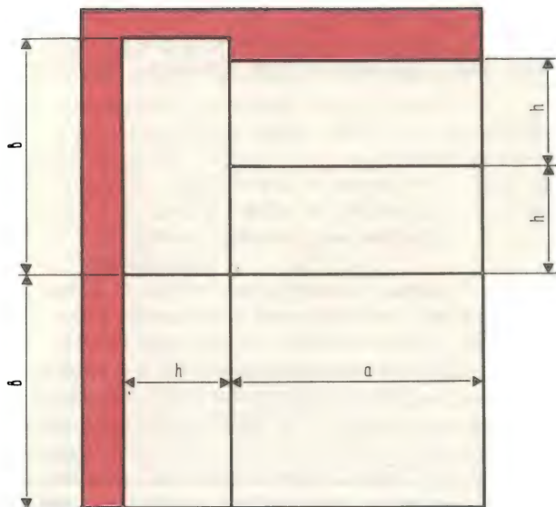
Рис. 21. Раскройка листа железа для изготовления бака
