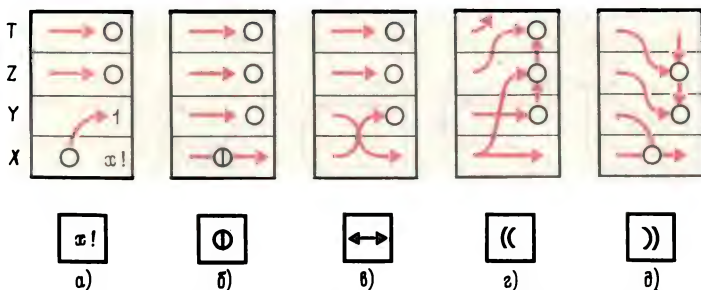
Рис. 7. Схемы работы операционного стека микрокалькулятора "Электроника БЗ-36"
