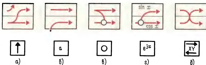
Рис. 8. Схемы работы операционного стека микрокалькулятора "Электроника БЗ-21"
