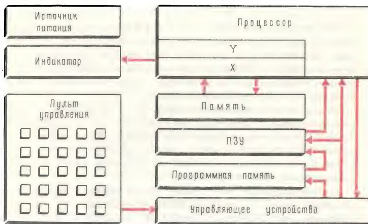
Рис. 5. Обобщенная схема микрокалькулятора
