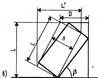
Рис. 27. "Протаскивание" шкафа с наклоном
