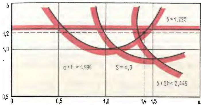
Рис. 20. Нелинейные ограничения в задаче об изготовлении бака
