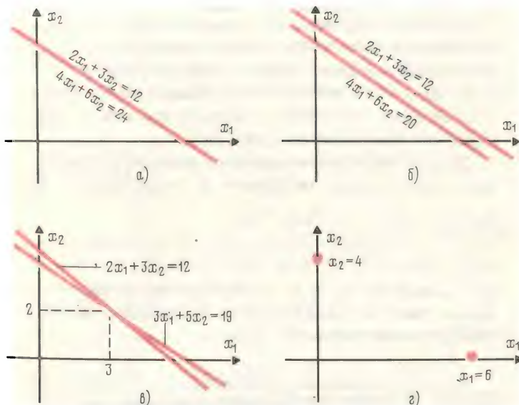
Рис. 17. Представление линейных уравнений на плоскости
