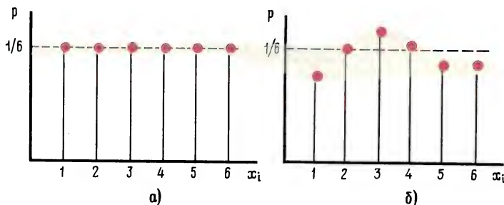
Рис. 18. Распределение вероятностей при бросании кубика
