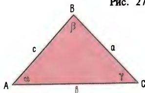
Рис. 28. Элементы треугольника
