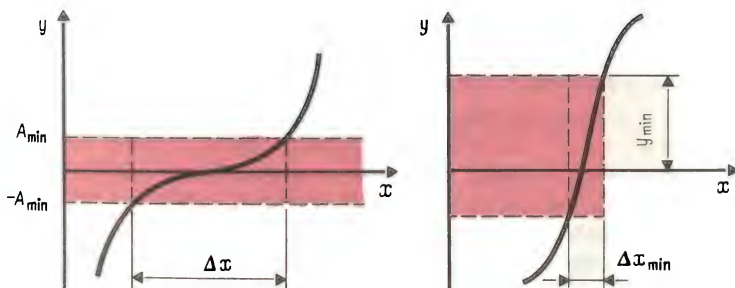
Рис. 15. Зависимость определения корня от поведения функции
