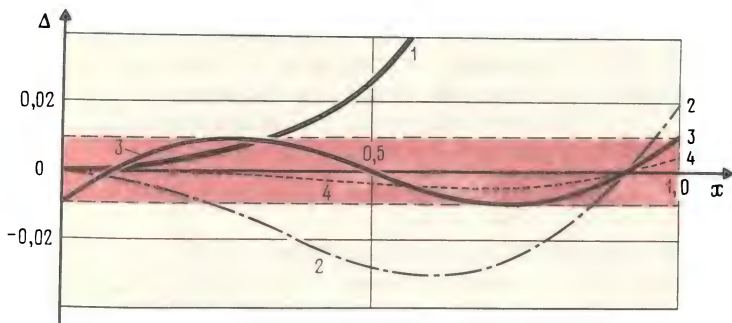
Рис. 12. Аппроксимации функции e^x
