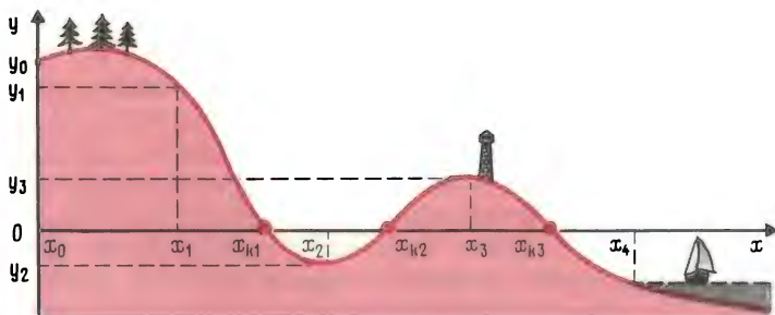
Рис. 13. Разрез местности по вертикали
