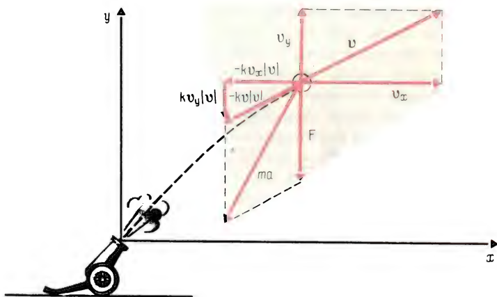
Рис. 36. Силы и скорости при полете снаряда
