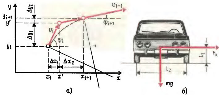
Рис. 38. Моделирование поворотов автомобиля
