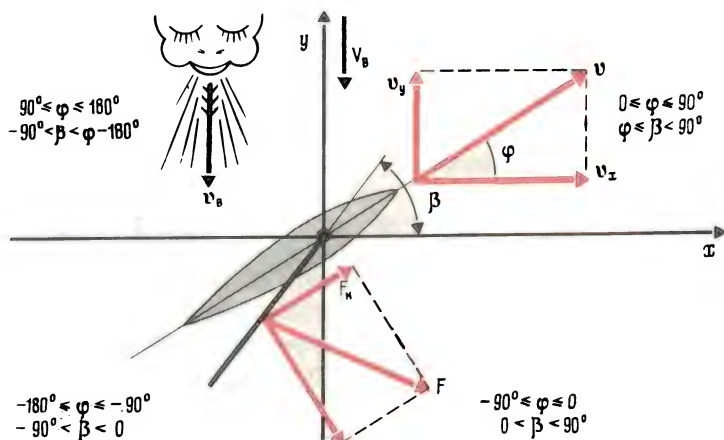
Рис. 34. Силы и скорости при движении яхты
