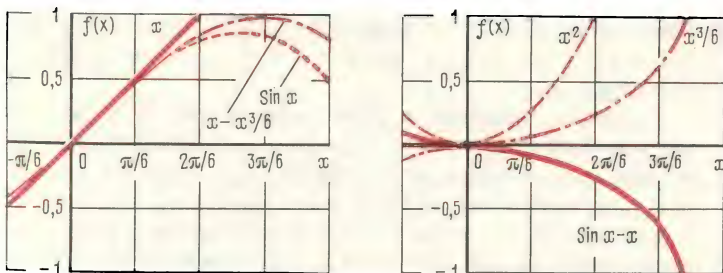
Рис. 11. Аппроксимации функции \sin x
