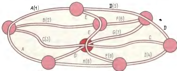
Рис. 48. Города и дороги
