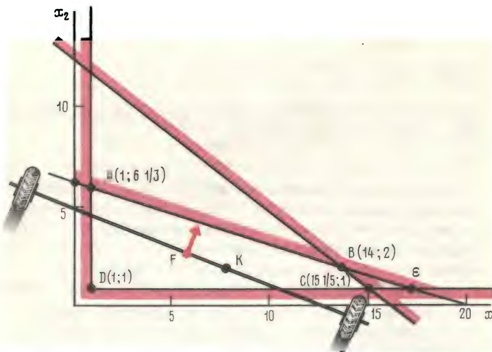
Рис. 24. Графическая модель в задаче о покупке мяса
