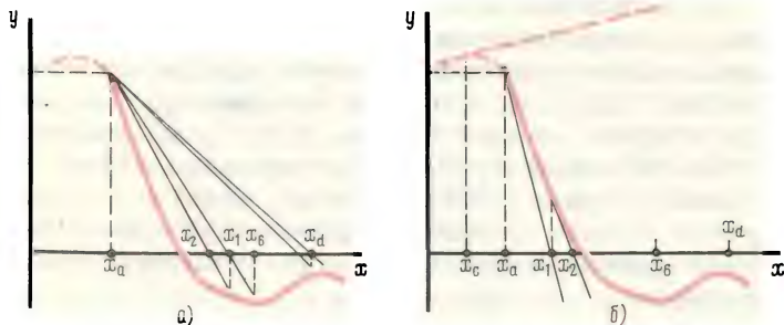
Рис. 16. Зависимость сходимости методов хорд и касательных от ширины исходного интервала
