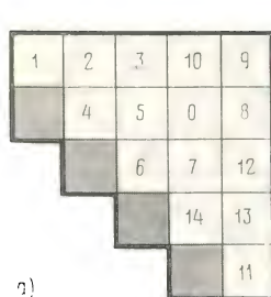
Рис. 50. Асим и Сим
